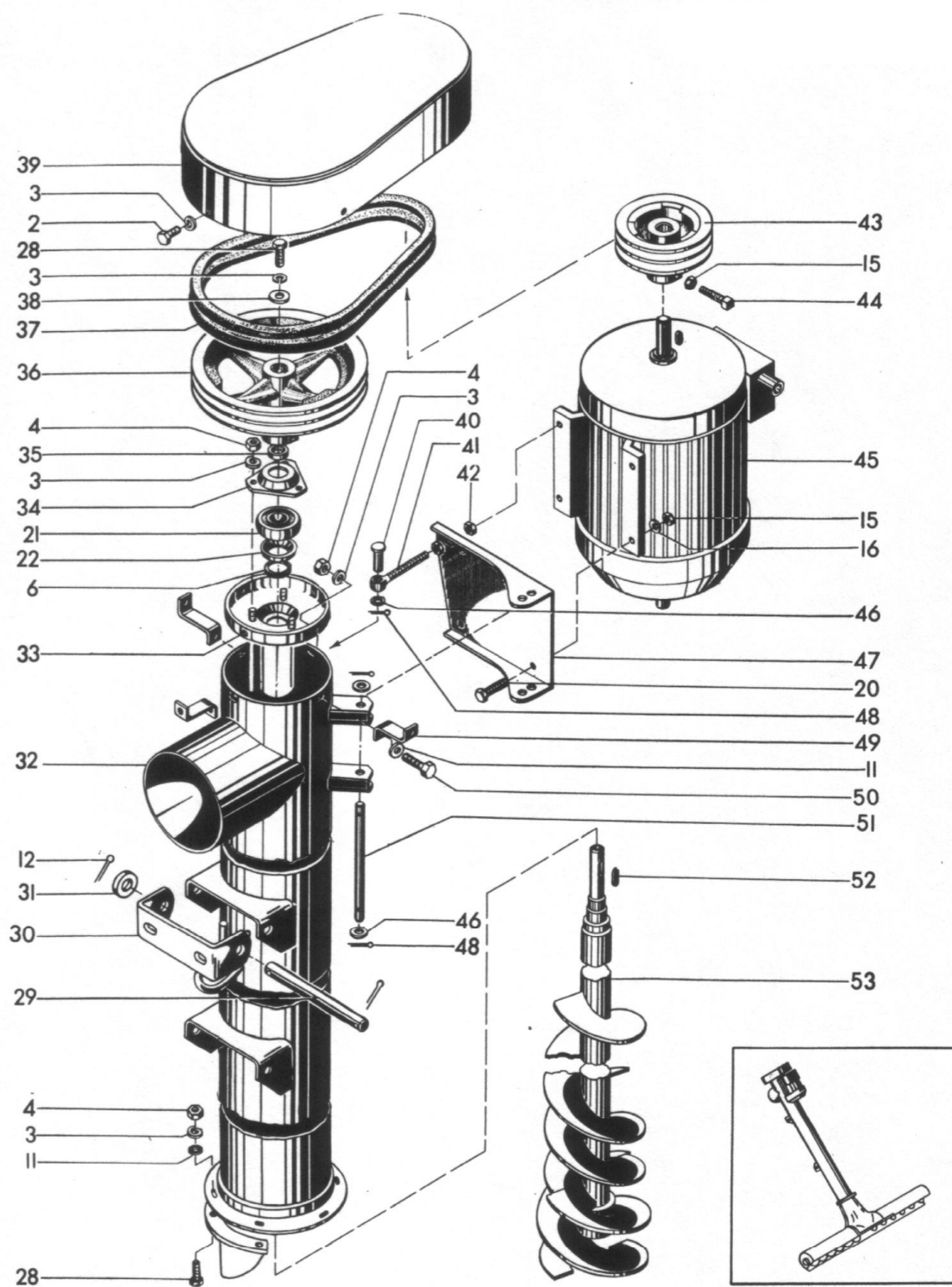
Рис.1 Устройство загрузочное ПС-10А.43.000 (верхняя часть)
